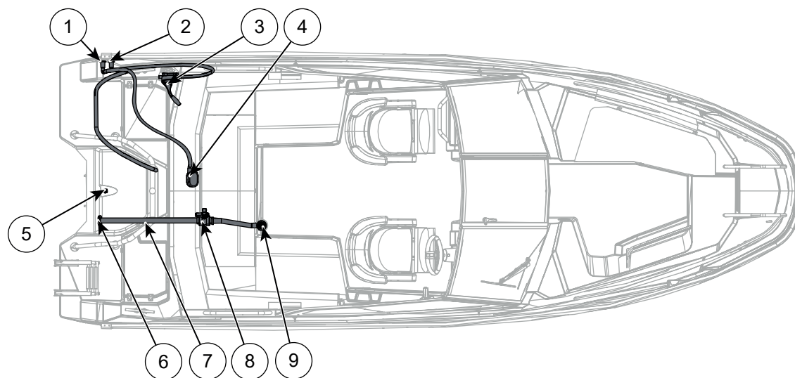
Figur 9.1 Cross 62 V MAX lensepumper og drenering
