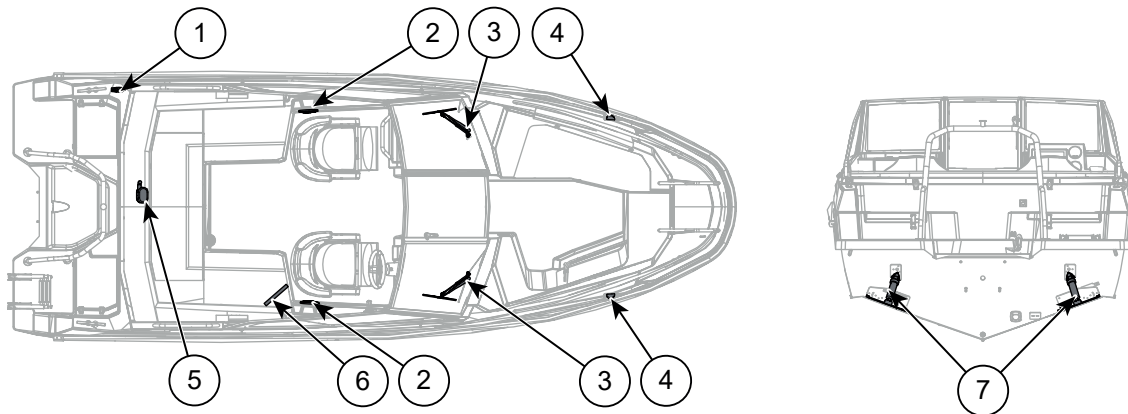
Figur 8.2 Cross 62 V MAX elektrisk utstyr
