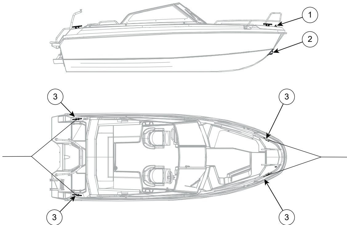
Figur 5.5 Cross 62 V MAX fortøynings- og slepepunkter
