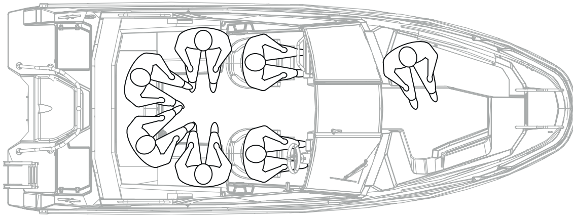
Figur 4.1 Cross 62 V MAX seter for maksimalt sju (7) passasjerer
