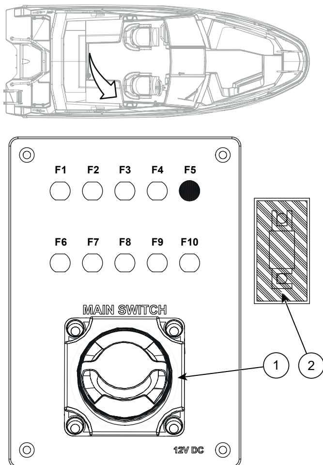
Figur 8.1 Cross 62 V MAX hovedbryter og sikringspanel
