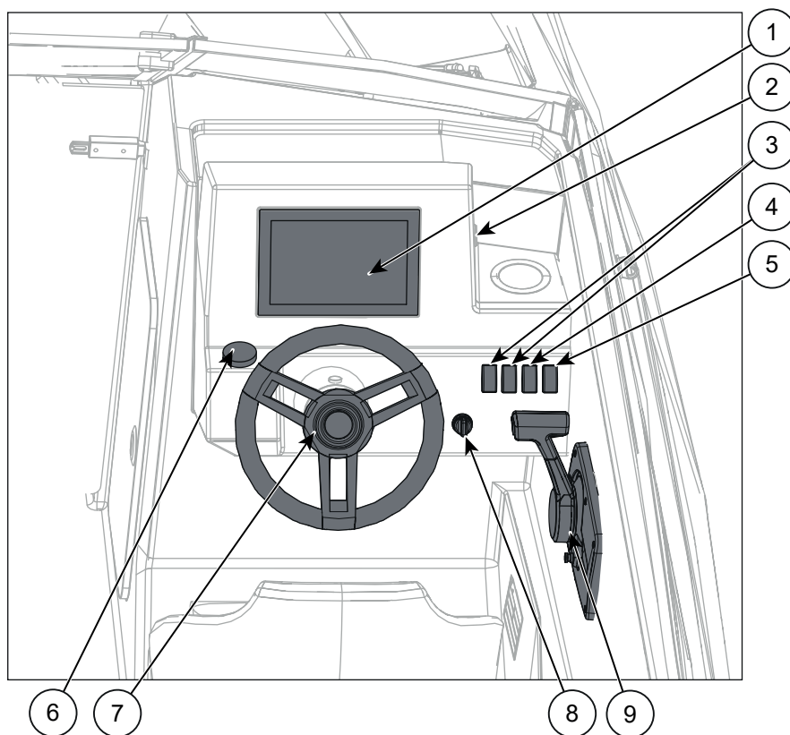
Figur 5.1 Cross 62 V MAX styrestasjonskontroller
